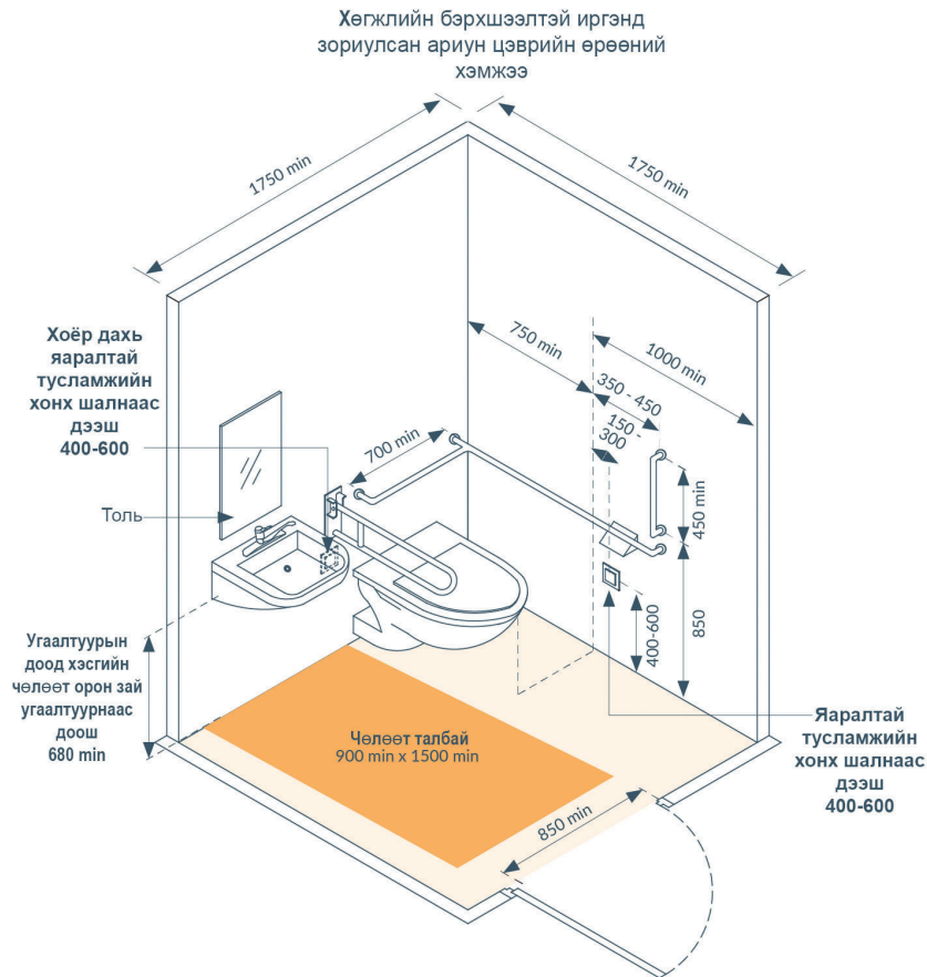
Зураг 33. Хөгжлийн бэрхшээлтэй иргэнд зориулсан ариун цэврийн өрөө (Жишээ зураг)
