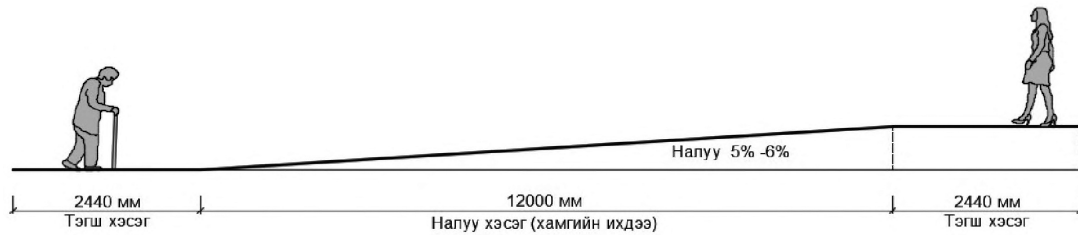
Зураг 22. Дагуу налуу, хөндлөн хэвгий (Жишээ зураг)
