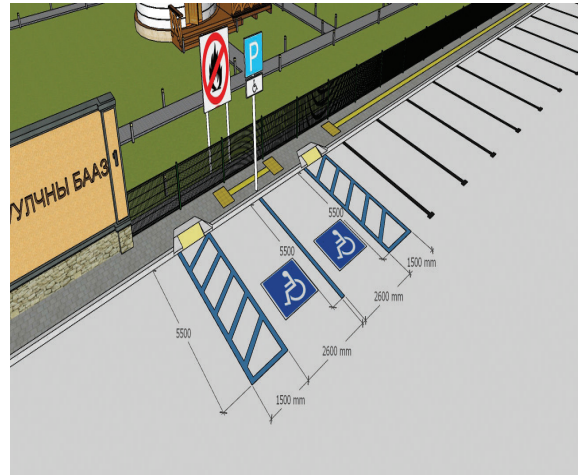
Зураг 6. Хөгжлийн бэрхшээлтэй иргэнд зориулсан тээврийн хэрэгслийн зогсоолын харагдах байдал (Жишээ зураг)
