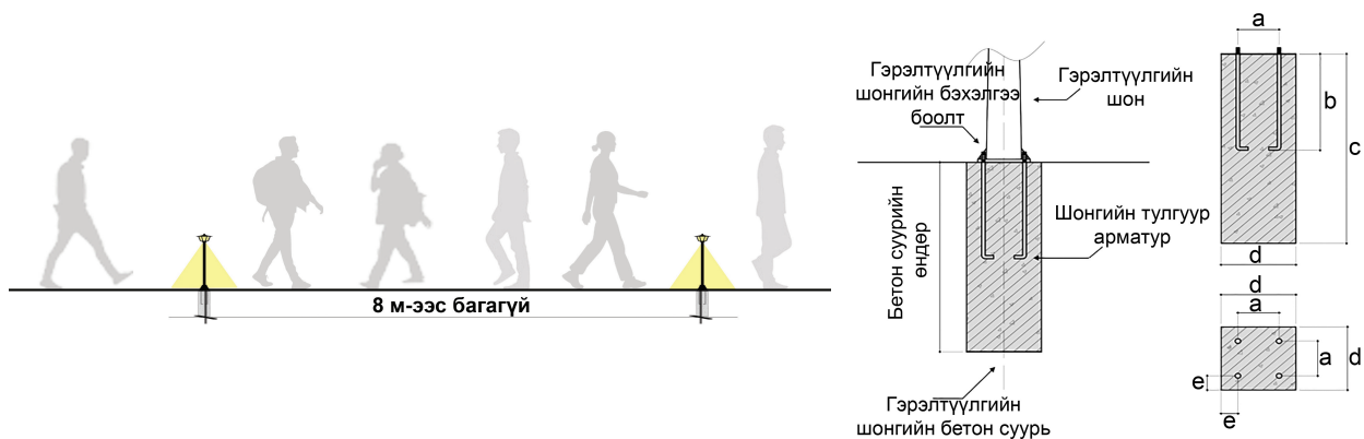
Зураг 23. Гэрэлтүүлэг хоорондын зай болон гэрлийг суурилуулах
